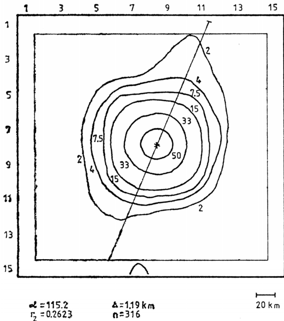
Abb. 3b: Glättungsmittelkarte der Fundverteilung der Abbildung 2a bei u = 3
