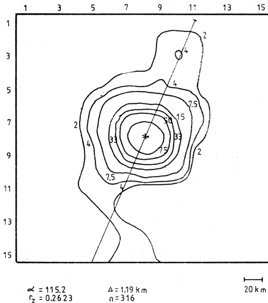
Abb. 3a: Glättungsmittelkarte der Fundverteilung der Abbildung 2a bei u = 2
