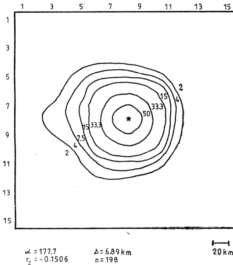
Abb. 5 Glättungsmittelkarte der Winterfunde von am Brutort beringten Hökerschwänen, Beringungsgebiet: ganze DDR, u = 3
