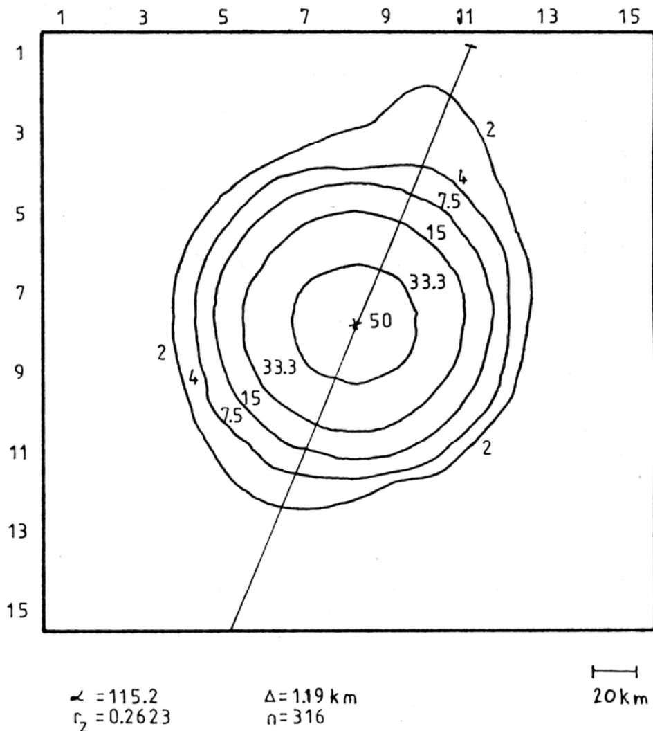
Abb. 3c: Glättungsmittelkarte der Fundverteilung der Abbildung 2a bei u = 4
