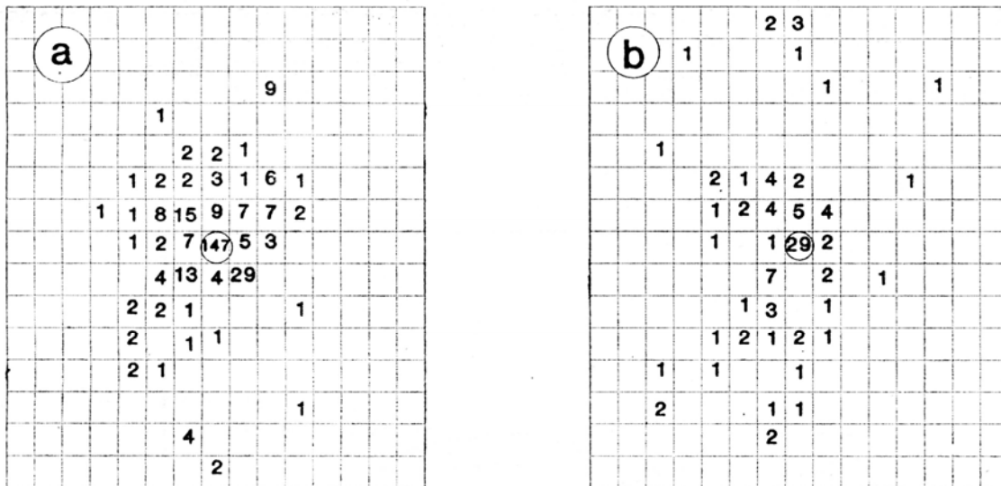
Abb. 2: Die Aufteilung der Lebendfunde von diesjährig im Bezirk Frankfurt/O. beringten Höckerschwänen auf 20 X 20-km-Rasterfelder rund um den Beringungsort; a: im I. Winter, b: in allen folgenden Brutzeiten
