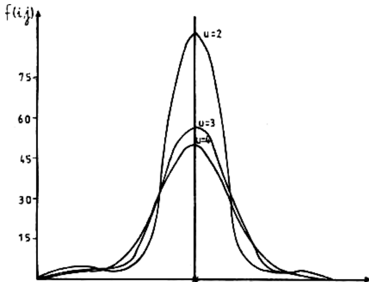
Abb. 4 f(i,j) -Profile entlang der in den Glättungsmittelkarten Abb. 3a-3c enthaltenen Schnittlinien (normierte Werte)
